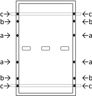
Schéma A3: Emplacement des trous de boulon
