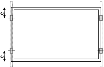
Schéma A2: Position de fixation par clip sur le côté court des cadres
