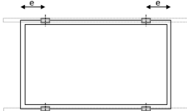
Schéma A2: Position de fixation par clip sur le côté long des cadres Rails de montage parallèles au cadre le plus long
