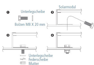
Abbildung 5. Komponenten für Schraubmontage
