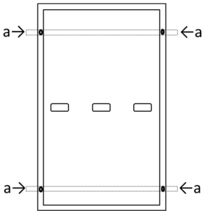
Bild B: Positionen der Montagel  cher f  r Schraubmontage
