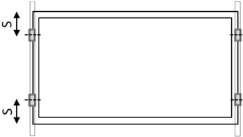
Schéma A2: Position de fixation par clip sur le côté court des cadres
