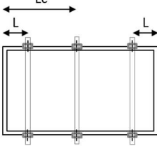
Schéma A1: Position de fixation par clip sur le côté long des cadres
