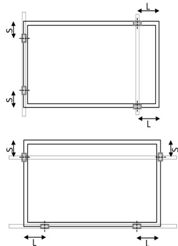
Schéma A3: Position de fixation par clip sur les côtés courts et longs des cadres
