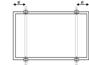
Schéma A1: Position de fixation par clip sur le côté long des cadres
