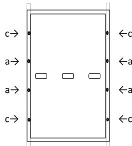
Schéma B2: Emplacement des trous de boulon
