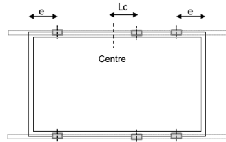
Schéma A2: Position de fixation par clip sur le côté long des cadres
