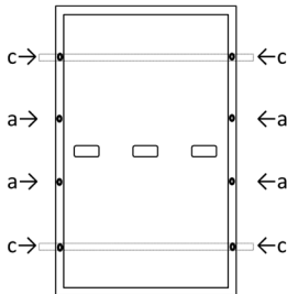
Schéma B1: Emplacement des trous de boulon
