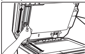
In einem Duplex Einzeldurchlauf-Einzug (DSPF)
