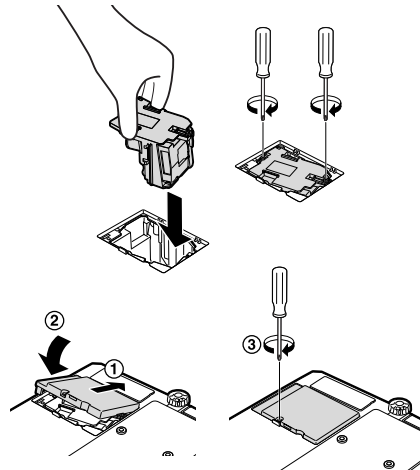
Befestigungsschrauben
