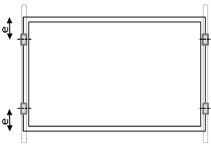
Schéma A1: Position de fixation par clip sur le côté long des cadres
