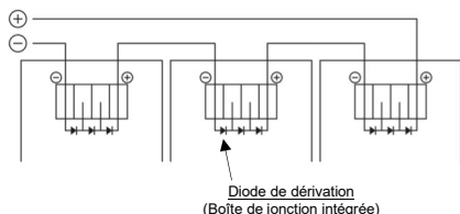
Figure 1. Série pour plus de tension
