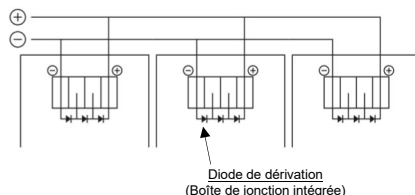
Figure 2. Parallèle pour plus de courant
