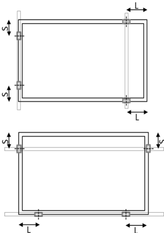
Schéma B: Position de fixation par clip sur les côtés courts et longs des cadres
