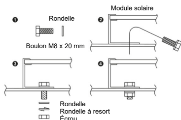
Schéma 2. Composants de montage par boulon et écrou
