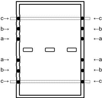
Schéma A3: Emplacement des trous de boulon
