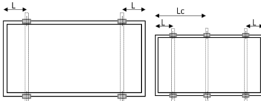
Bild A1: Klemmen an langer Rahmenseite
