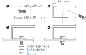
Klemmen an langer &amp; kurzer Rahmenseite
