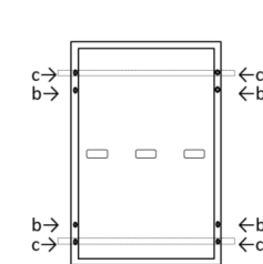
Bild A3: Positionen Montagelöcher
