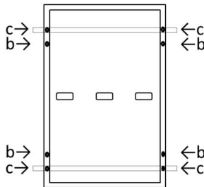
Schéma A3: Emplacement des trous de boulon
