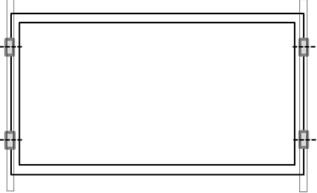
Schéma A2: Position de fixation par clip sur le côté court des cadres
