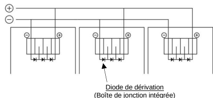
Figure 2. Parallèle pour plus de courant
