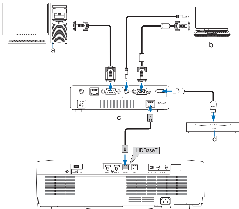
a: Υπολογιστής (για χρήση ελέγχου) / b: Υπολογιστής (για χρήση εξόδου) / c: Παράδειγμα συσκευής μετάδοσης / d: Συσκευή βίντεο εξόδου HDMI
