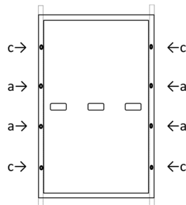
Bild B2: Positionen der Montagelöcher für Schraubmontage Montageschienen parallel zur langen Rahmenseite
