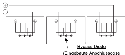
Abb. 1. Reihenschaltung zur Erhöhung der Spannung
