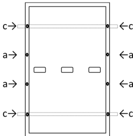
Schéma B1: Emplacement des trous de boulon Rails de montage perpendiculaires au cadre le plus long
