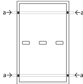
Bild A3: Positionen der Montagelöcher für Schraubmontage
