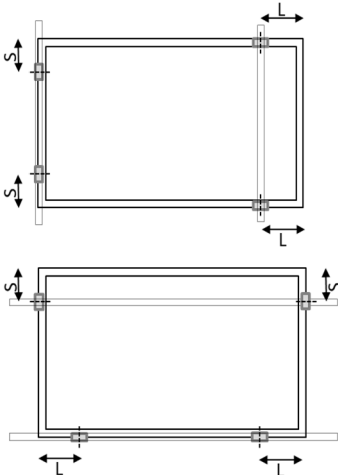
Bild B: Klemmenpositionen an langer und kurzer Rahmenseite
