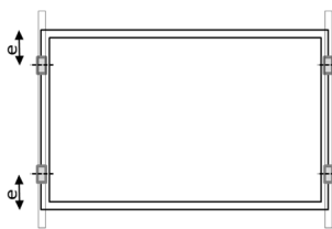
Schéma A2: Position de fixation par clip sur le côté court des cadres
