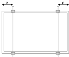
Schéma A1: Position de fixation par clip sur le côté long des cadres
