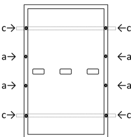
Bild B1: Positionen der Montagelöcher für Schraubmontage Montageschienen quer zur langen Rahmenseite
