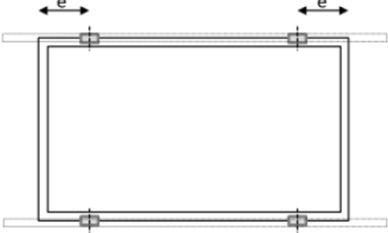
Bild A2: Klemmenposition an langer Rahmenseite Montageschienen parallel zur langen Rahmenseite
