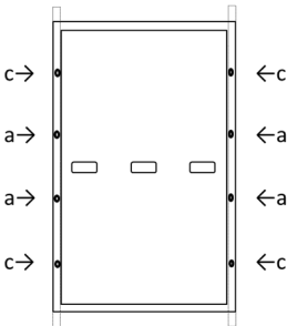
Bild B2: Positionen der Montagelöcher für Schraubmontage Montageschienen parallel zur langen Rahmenseite
