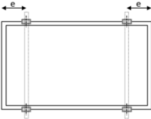
Bild A1: Klemmenposition an langer Rahmenseite Montageschienen quer zur langen Rahmenseite
