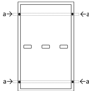
Bild A3: Positionen der Montagelöcher für Schraubmontage
