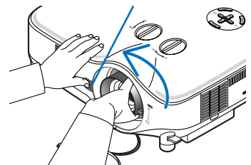
Botón LENS RELEASE
