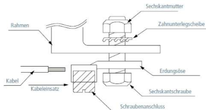
ABBILDUNG 3. BEISPIEL FÜR EINEN MÖGLICHEN ERDSCHLUSS
