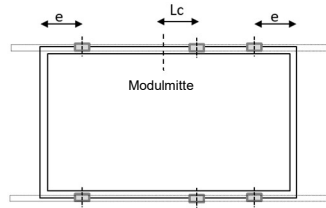
Bild A2: Klemmenposition an langer Rahmenseite
