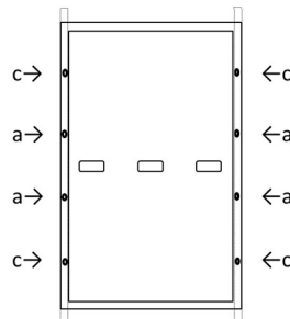
Bild B2: Positionen der Montagelöcher für Schraubmontage
