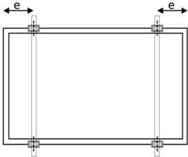
Bild A1: Klemmenposition an langer Rahmenseite
