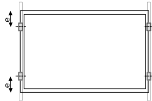
Bild A2: Klemmenposition an kurzer Rahmenseite
