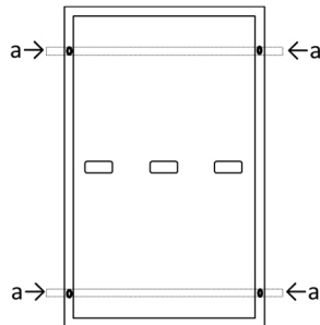
Bild B: Positionen der Montagelöcher für Schraubmontage
