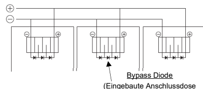
Abb. 2. Parallelschaltung zur Erhöhung der Stromstärke
