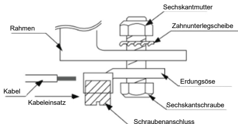
Abb. 3. Beispiel für einen möglichen Erdanschluss
