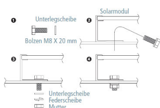
Abbildung 5. Komponenten für Schraubmontage
