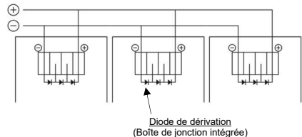
Schéma 2. Parallèle pour plus de courant
